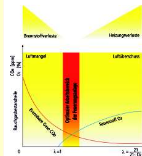
Verbrennungs-Optimierungs-Diagramm:
